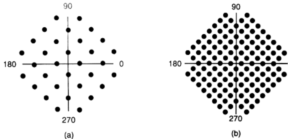
(a) V.32 szabvány 9600 b/s-hoz. (b) V.32 bis szabvány 14 400 b/s-hoz
